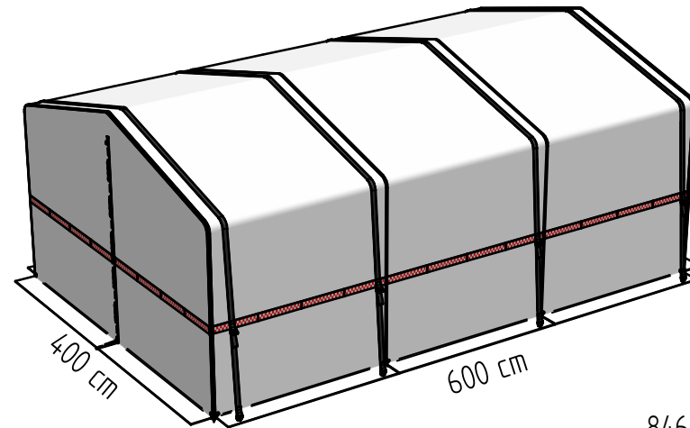
846915.400600 L = 600 cm
