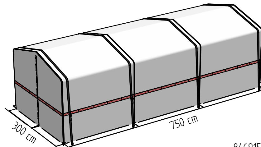
846915.300750 L = 750 cm
